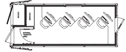
MWD Cabin
